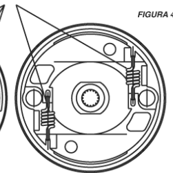
MOLLE DA SOSTITUIRE - SPRINGS TO BE REPLACED RESSORTS À REMPLACER - ZU ERSETZENDE FEDER MUELLES PARA SUSTITUCIÓN
