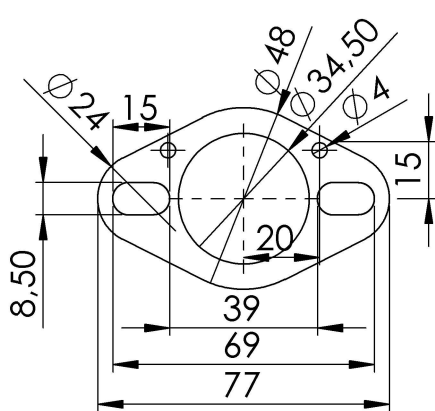
S.s. flange Cod.206443R
